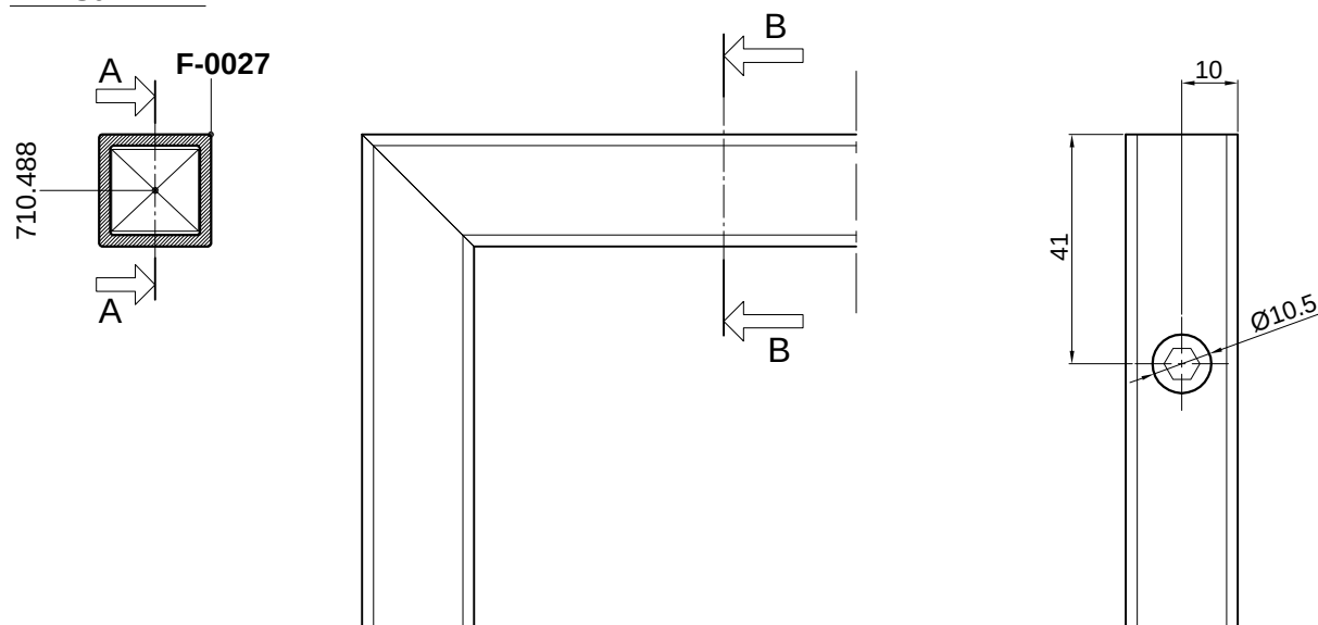
PRESJEK B-B
